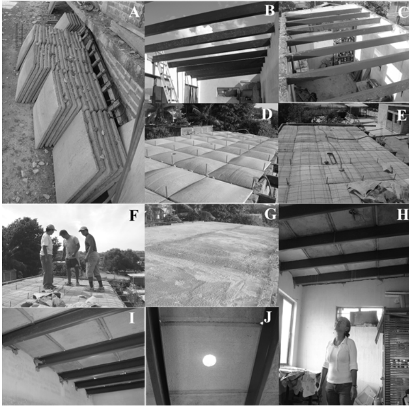
Figura 7.3. Proceso de construcción de techo Domozed, de la foto A hasta la foto J, se observa el proceso sucesivo de fabricación del techo.
