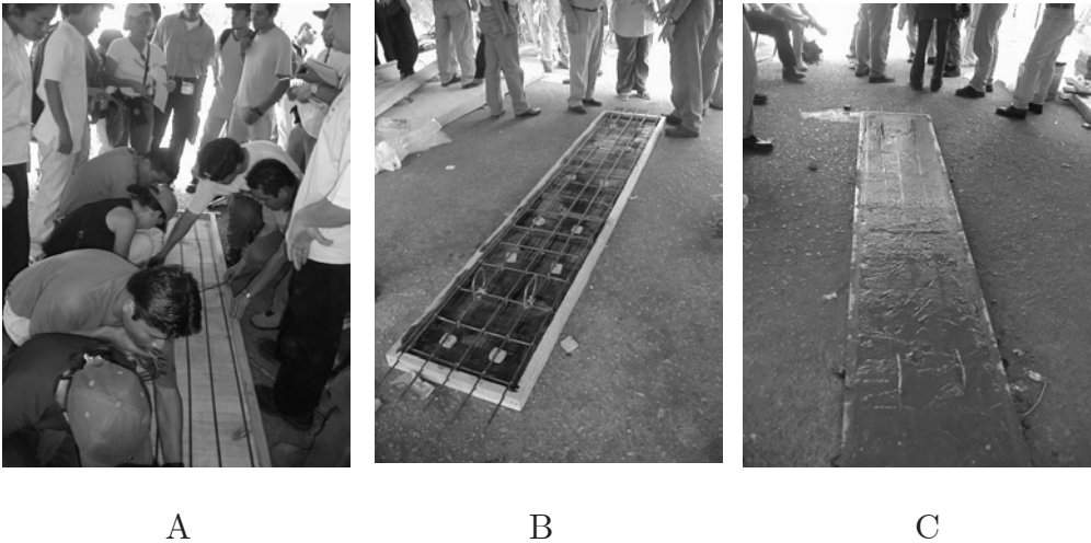
Figura 1.23. Tecnologías presentadas en el Taller de Transferencia de Tecnología de Chiapas. En las fotos A - C se muestra el proceso de fabricación de pre – losa de concreto.
