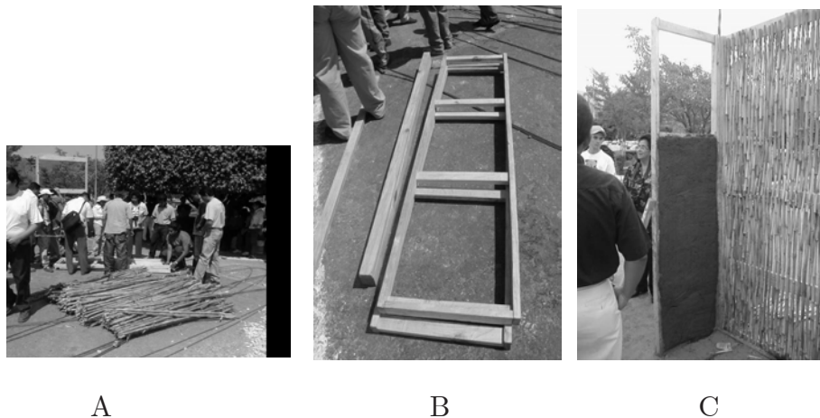
Figura 1.17. Tecnologías presentadas en el Taller de Transferencia de Tecnología de Chiapas. En la foto A muestra en el tallo del maíz utilizado para estructurar el panel de Quincha, en la foto B, estructura del panel de Quincha. En la foto C, Panel de Quincha prefabricado.
