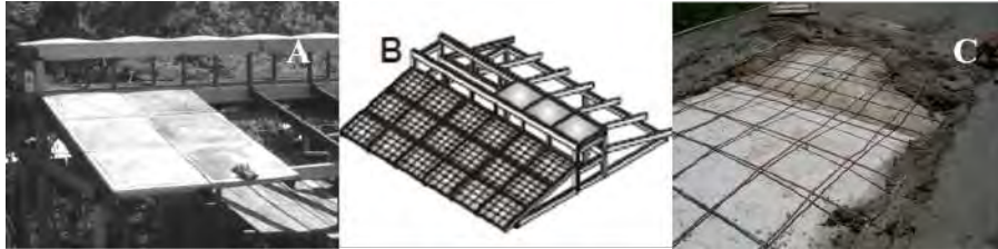
Figura 3.22. Refuerzo de acero con malla electrosoldada en la capa de compresión sobre Domotej
