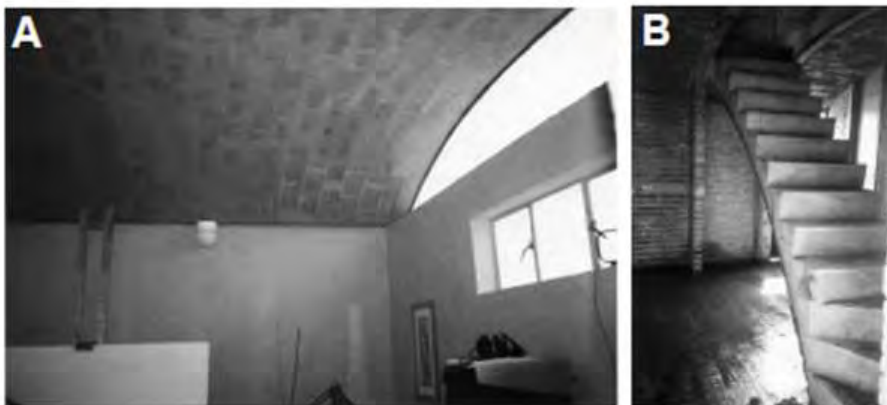
Figura 2.11-. Bóvedas de ladrillo, Arq. Mario Larrondo. Foto A y B, Vivienda en la Ciudad de México D. F.
